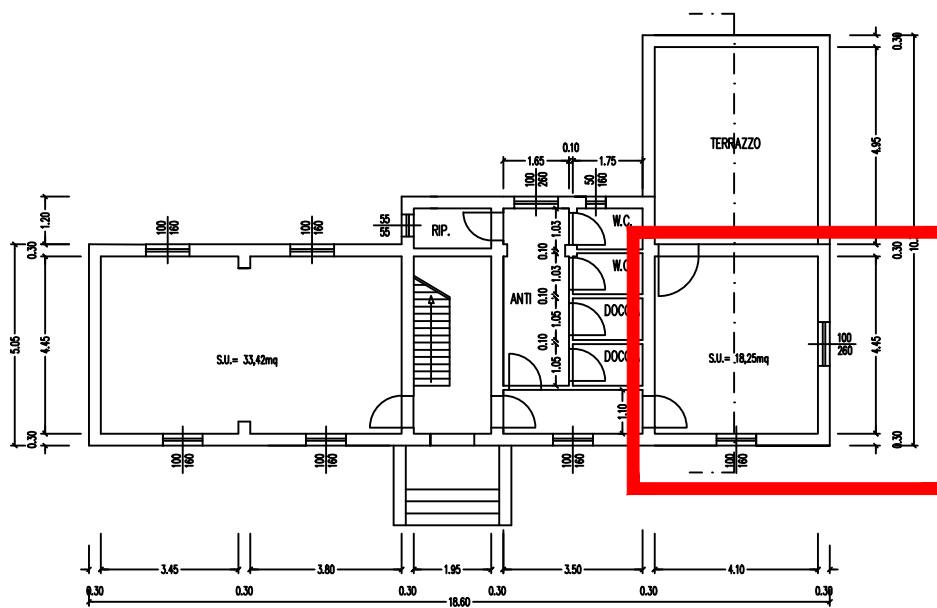
PIANO RIALZATO Scala 1:100
